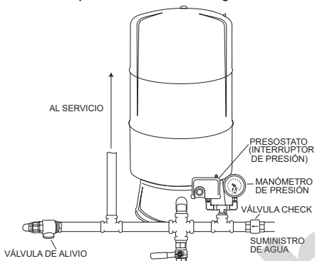
Instalación típica de una bomba sumergible
